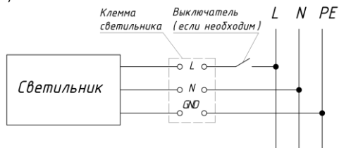
Рисунок 8. Подключение светильника к сети \sim 220V .
