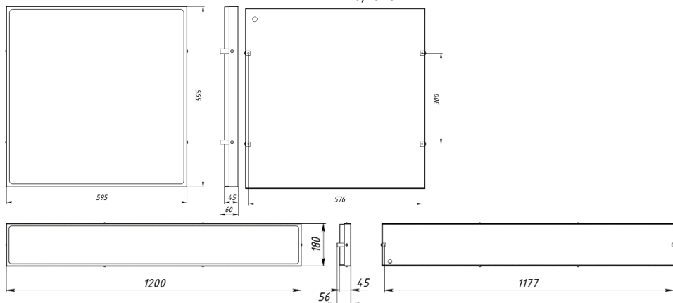
Рисунок 6 – Варианты светильников Офис 595x595 IP54 и ЛПО 1200x180 IP54 с уголком для накладного монтажа.
