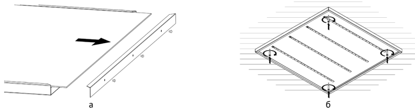
Рисунок 5 — Накладной монтаж светильника Geniled серии Офис, ЛПО.
