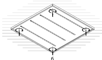
Рисунок 5 — Накладной монтаж светильника Geniled серии Офис, ЛПО.
