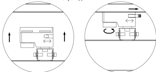
Рисунок 10. Крепление на шинномпроводе.
